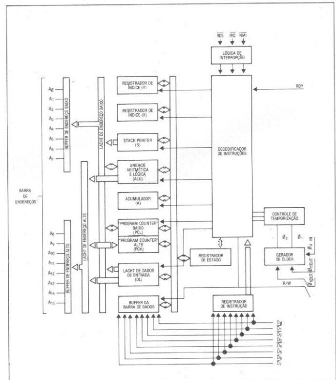
Figura 1 — Diagrama de blocos do microprocessador 6502
